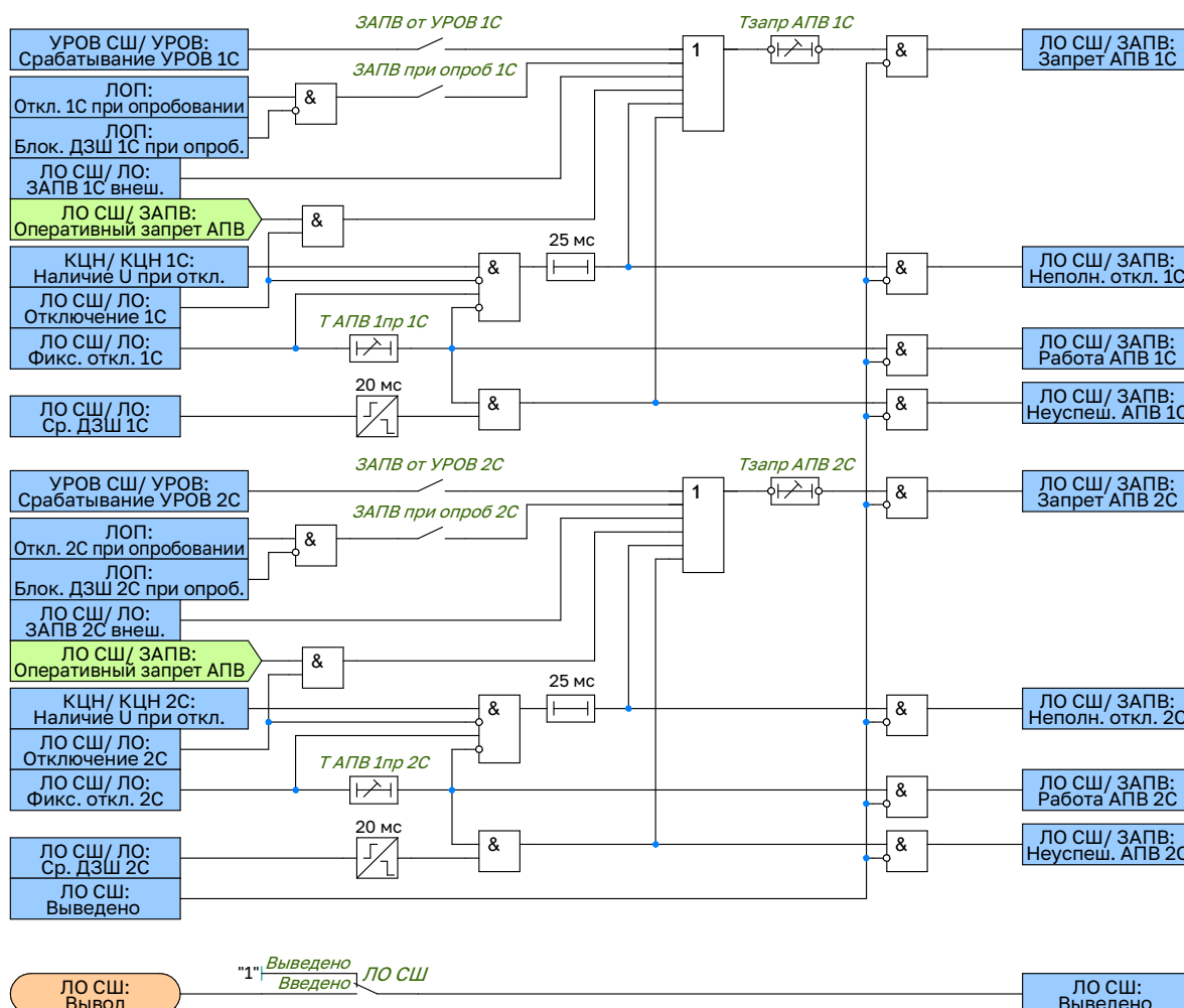
ЗАПВ (Логика запрета АПВ) 7751
