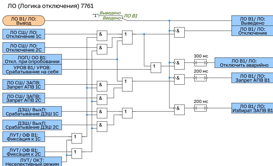
Рисунок 2.16 – Функциональная схема логики отключения выключателя В1
