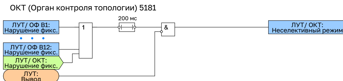
Рисунок 2.7 – Функциональная схема логики нарушения фиксации
